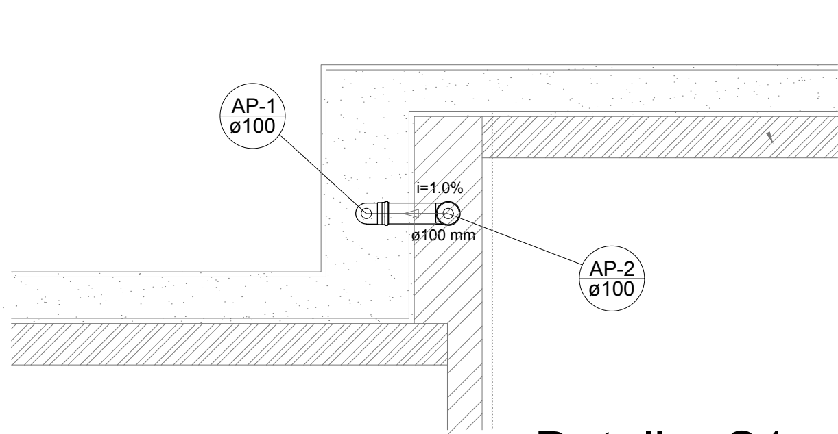
Detalhe S1 escala 1:25
